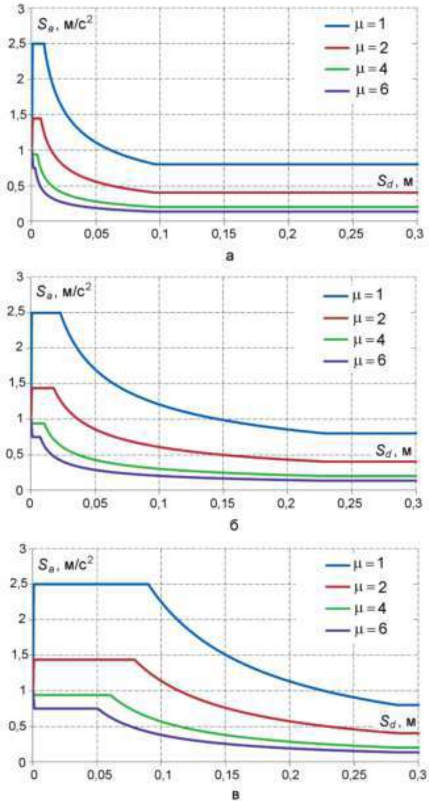
Рисунок Д.2 – Графіки " S_a - S_d " за сейсмічних впливів інтенсивністю 7 балів і різних коефіцієнтах податливості \mu будівлі (споруди)
